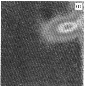
图3 四级线圈电流为 25.1 A 时,第一组线圈组合的四极磁阱向 QUIC 磁阱的转变过程 (a),(c),(e)为数值模拟结果(曲线)与实验结果(数据点)的对比;(b),(d),(f)为与(a),(c),(e)相应的原子吸收成像照片. Ioffe 线圈的电流从上而下分别为 0, 16.6 和 18 A. 相对于(a)图,(c)和(e)的成像系统分别移动了约 8 和 11 mm
