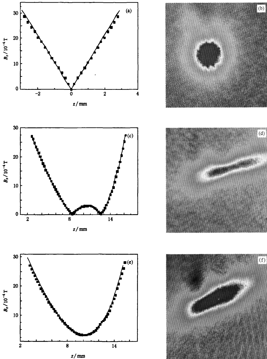
图 4 四极线圈电流为 25.1 A 时,第二组线圈组合的四极磁阱向 QUIC 磁阱的转变过程 (a),(c),(e)为数值模拟结果(曲线)与实验结果(数据点)的对比;(b),(d),(f)为与(a),(c),(e)相应的原子吸收成像照片.Ioffe 线圈的电流从上而下分别为 0,33 和 35 A.相对于(a)图,(c)和(e)的成像系统分别移动了约 7 和 9 mm
